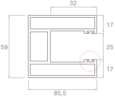
■ 308207 GUÍA AL GSR - 66 GSR-66 ALU GUIDE COULISSE ALU GSR-66
