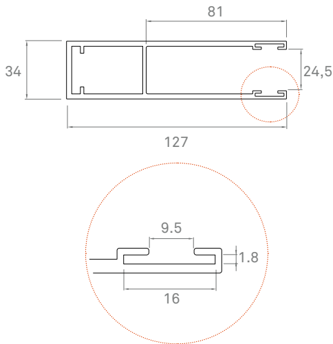
■ 308205 GUÍA AL GS-130 GS-130 ALU GUIDE COULISSE ALU GS-130
