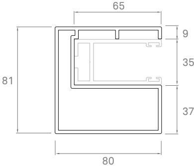
■ 308223 GUÍA AL PREMARCO 80 X 80 ALU FRAME GUIDE 80 X 80 COULISSE ALU CADRE 80 X 80
